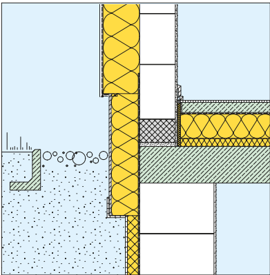
Sockeldetail mit einem KS-ISO-Kimmstein am Wandfuß.
