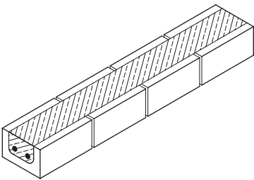
KS-Sichtmauersturz Höhe 113
